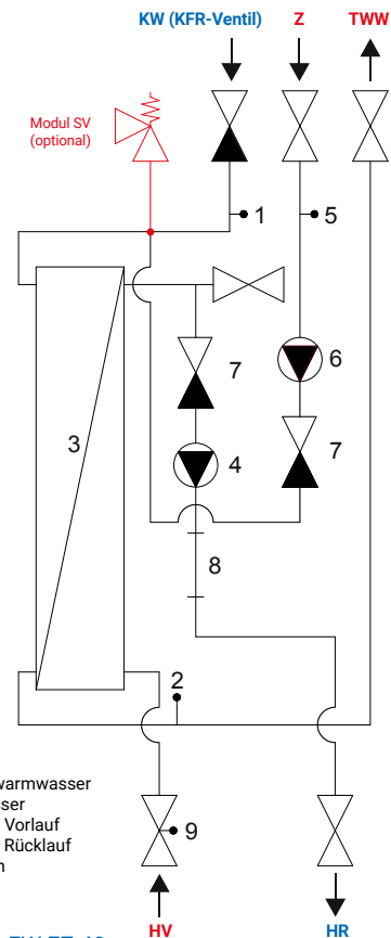
Abbild: FW-EZ 40
