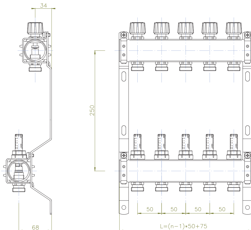
L = Länge des Verteilers n = Anzahl der Heizkreise
