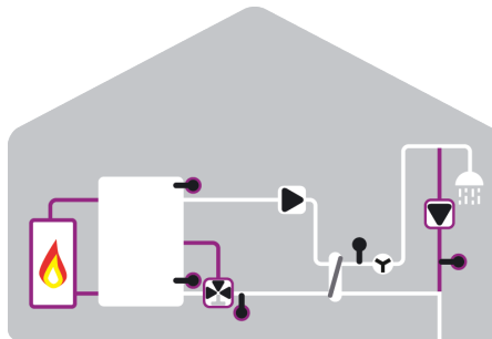
Zusatzfunktion Zirkulation, Speicherschichtung und Speicheraufheizung S1 Zirkulation S6 RL Primär S4 Speicher oben S7 VFS S5 Speicher unten
