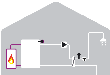
Zusatzfunktion Speicheraufheizung S4 Speicher oben S7 VFS
