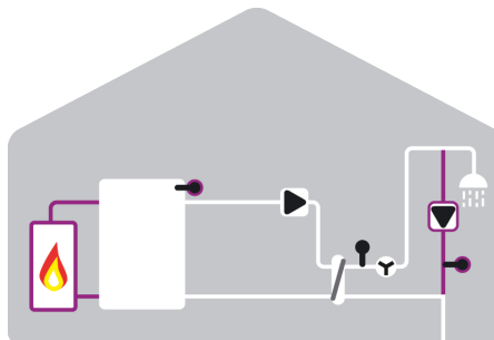
Zusatzfunktion Speicheraufheizung und Zirkulation S1 Zirkulation S7 VFS S4 Speicher oben
